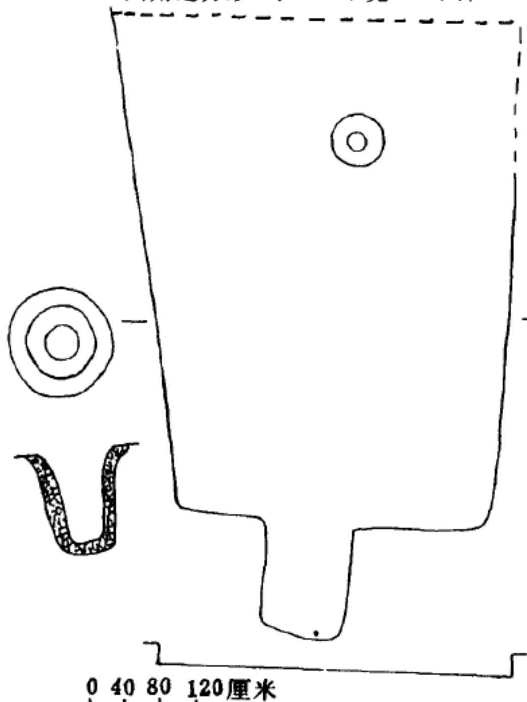
图一〇 AF9 平剖、面图
