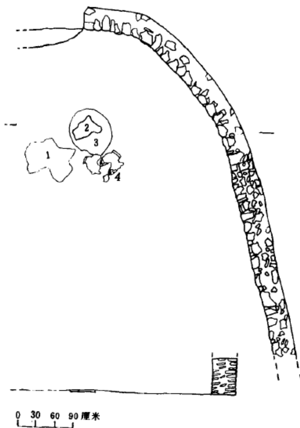
图九 AF2平、剖面图
