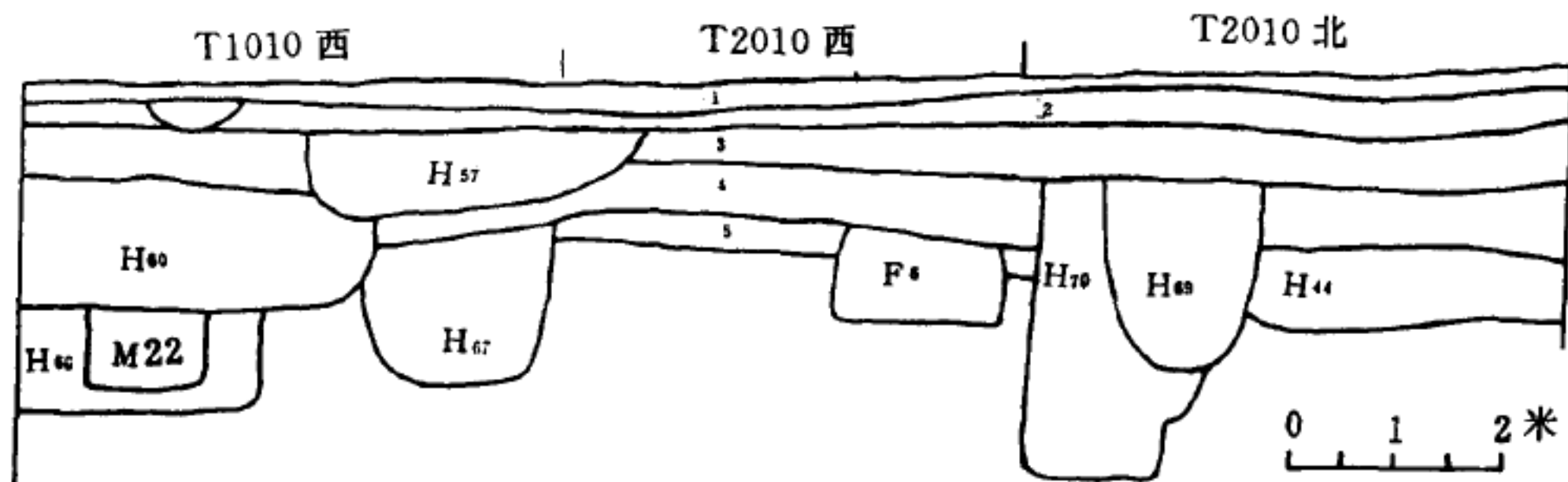
图二 地层剖面图
