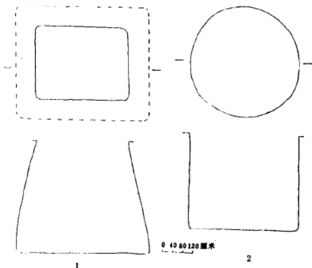
图四 窖穴平、剖面图 1. AH14 2. AH16
