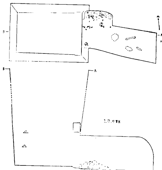
图八 83凤八西M7平、剖面图
