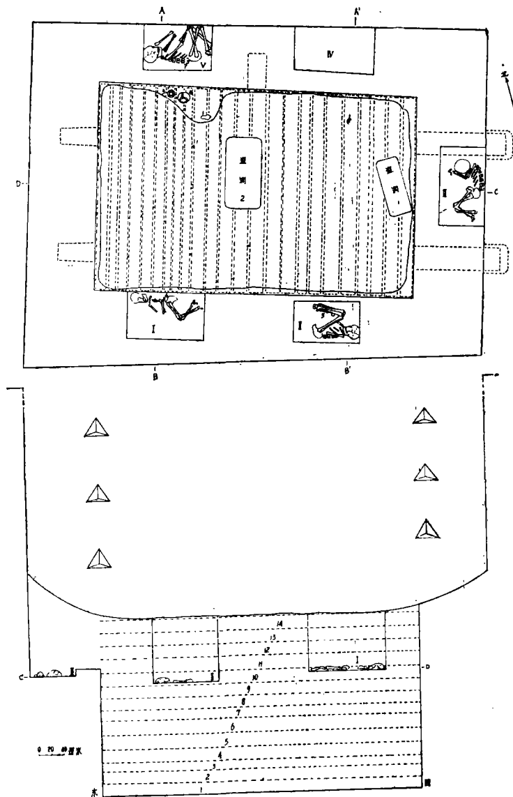
图四：a 83凤八西M3平、剖面（南视）图
