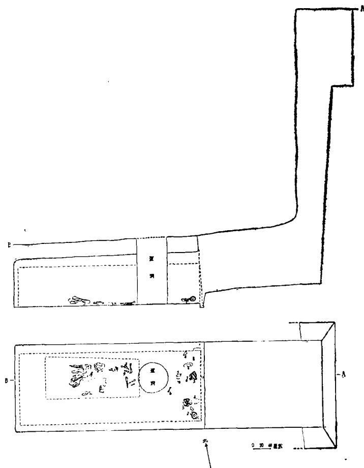
图九 83凤八西M2平、剖面图
