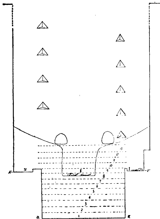
图四: b 83凤八西M3横剖面(东视)图
