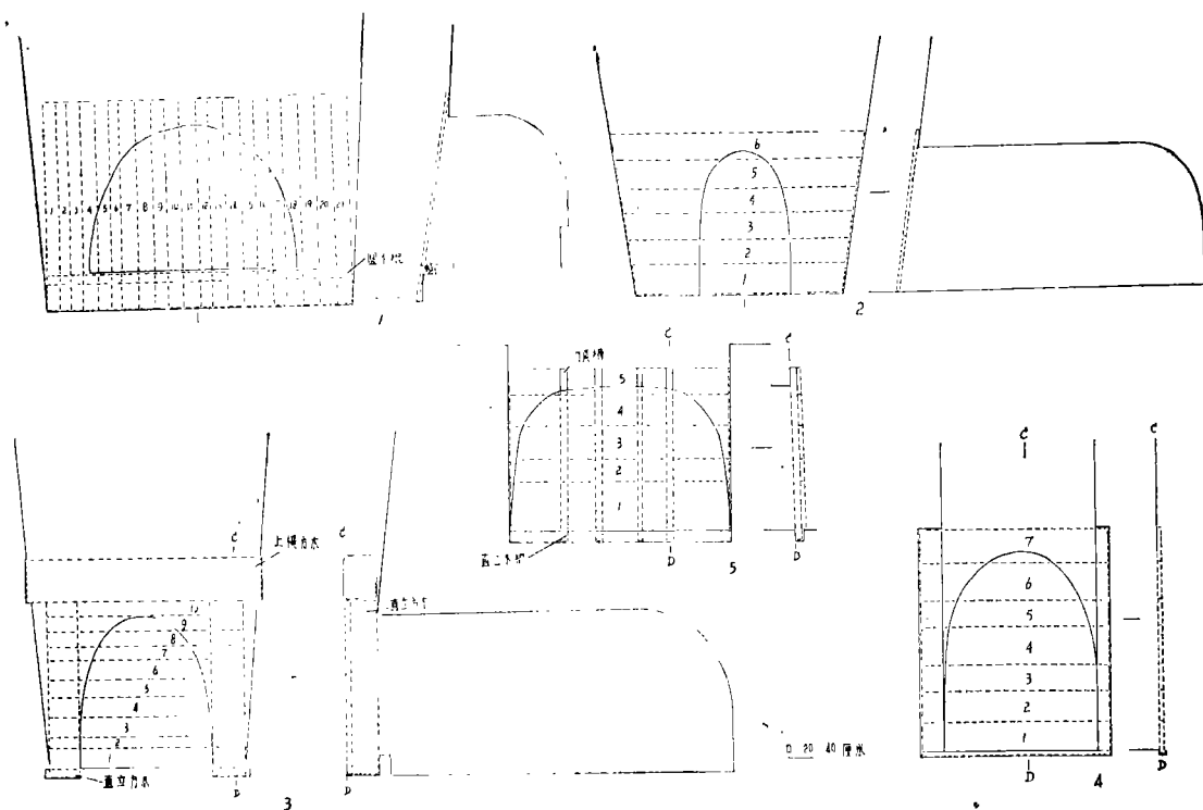
图三 洞式墓封门构筑方法
