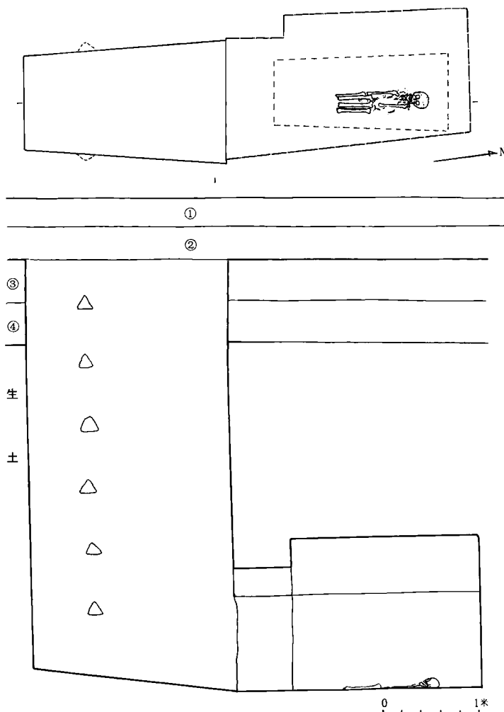
图十一 M7平剖面图
