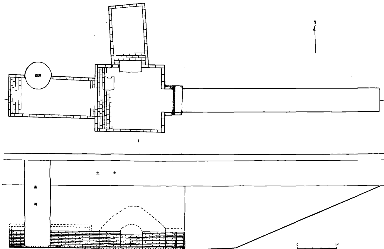
图八 M6剖面图
