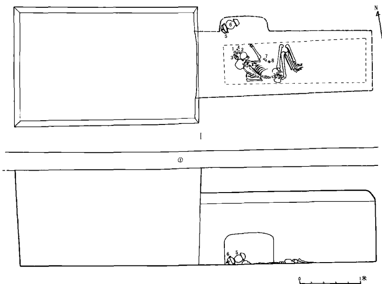
图四 M3剖面图
