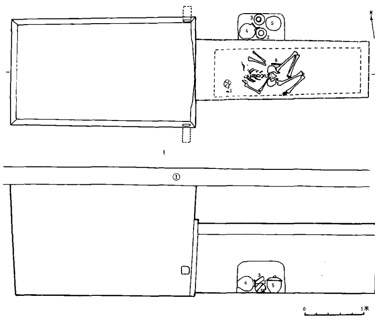
图五 M5剖面图
