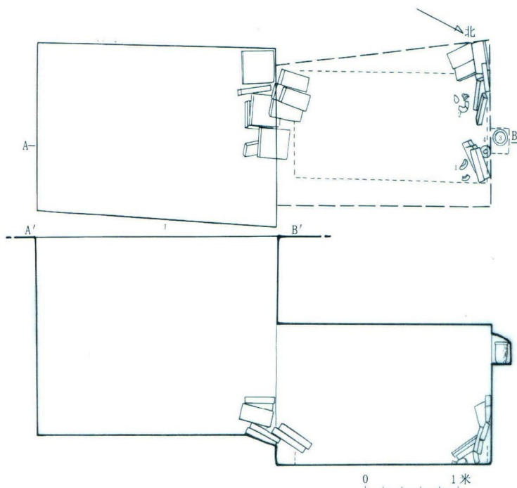
图六 M142墓葬剖面图
