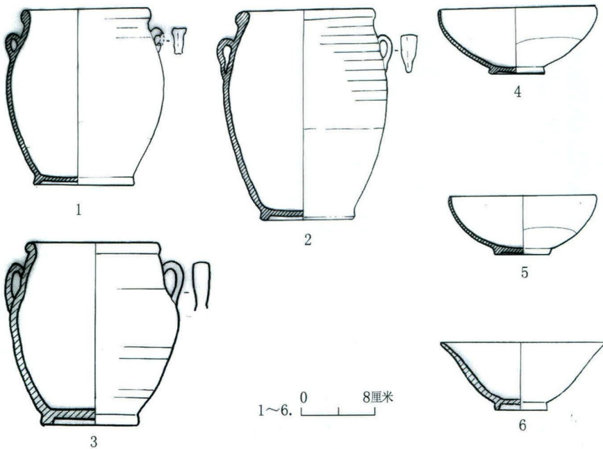
图八 M141、M142、M179出土瓷罐、瓷碗 1~3. 瓷罐（M141：1、M142：3、M179：1） 4~6. 瓷碗（M142：2、M142：1、M151：2）
