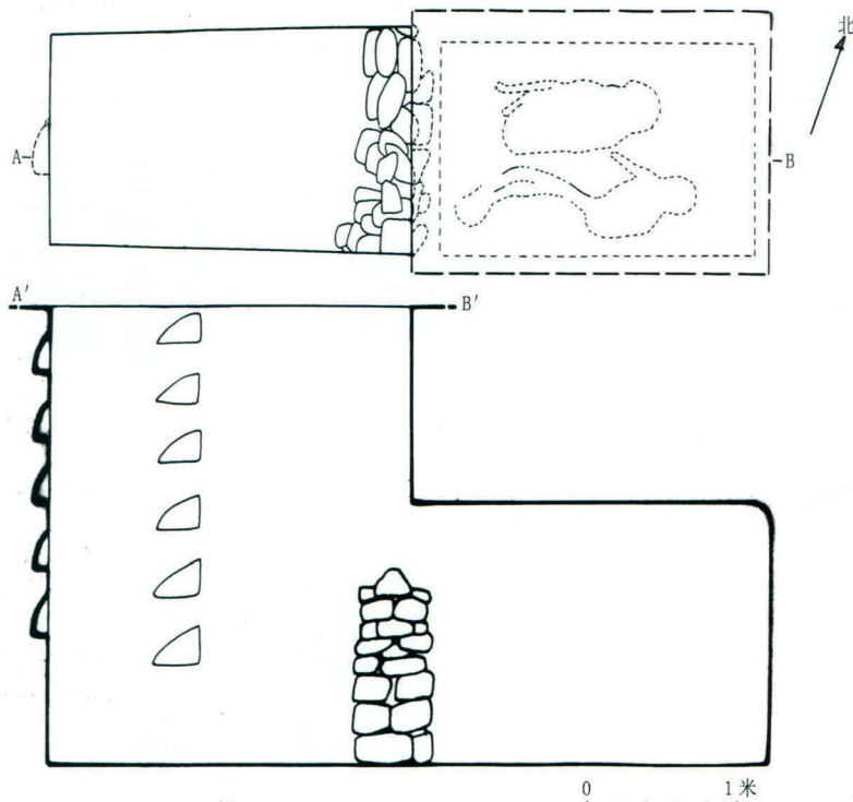
图七 M178墓葬剖面图
