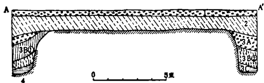
图六 凤南Ⅲ号秦陵园T2横剖面图
