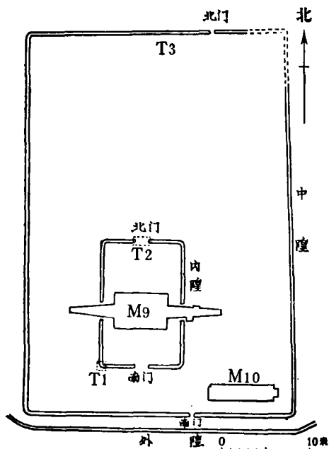
图三 凤南Ⅲ号秦公陵园内、中隍平面示意图
