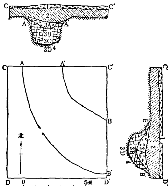
图四 凤南Ⅲ号秦公陵园T1剖面图
