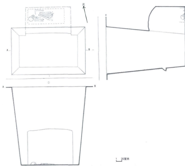
图六 六道村M3平剖面图
