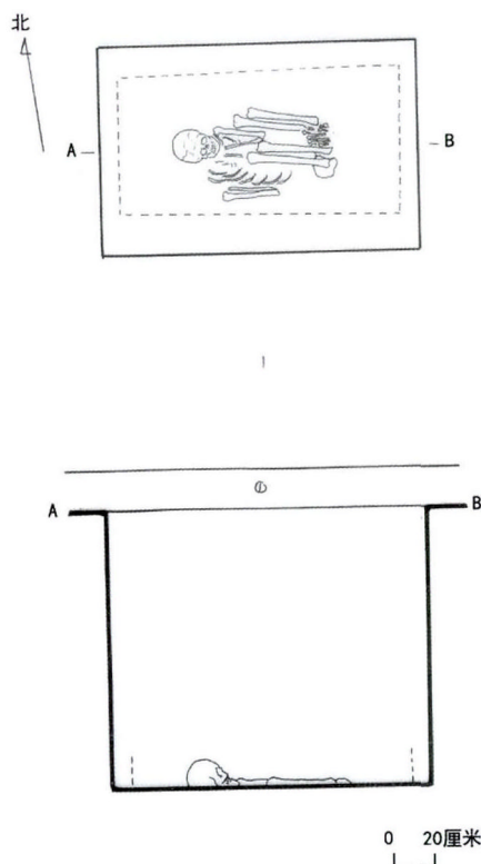
图三 六道村M26平剖面图
