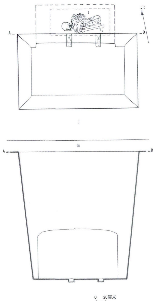
图十 六道村M15平剖面图
