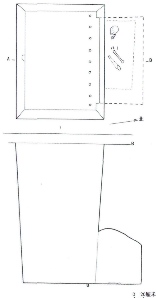
图九 六道村M21平剖面图
