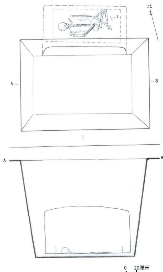
图七 六道村M20平剖面图
