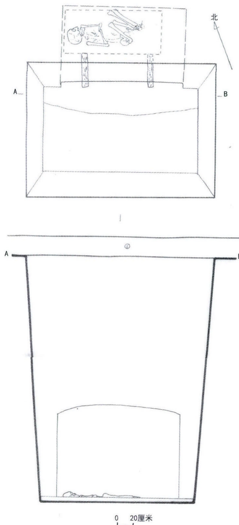
图八 六道村M4平面图
